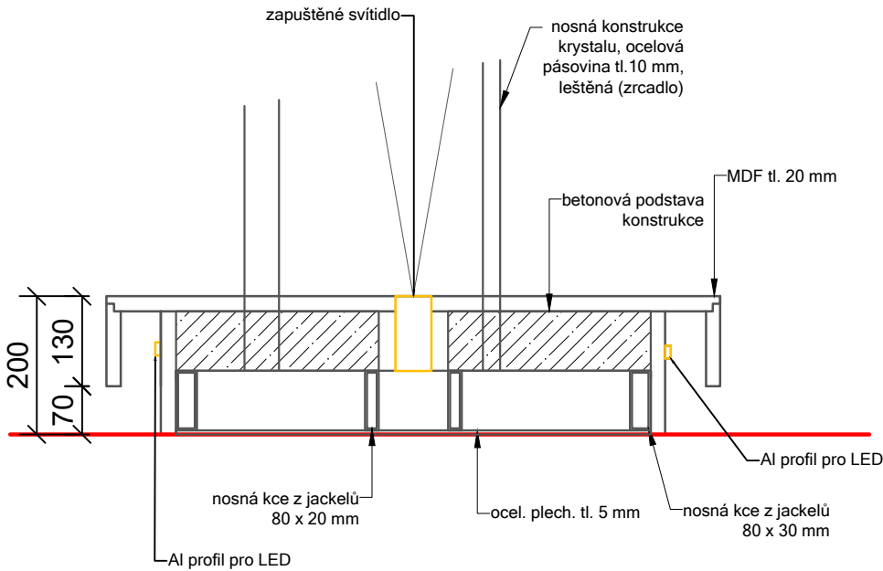
ŘEZ SOKLEM M 1:100
